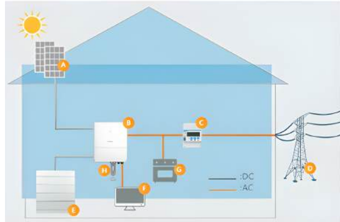
SƠ ĐỒ NGUYÊN LÝ HOẠT ĐỘNG HỆ THỐNG ĐIỆN MẶT TRỜI
